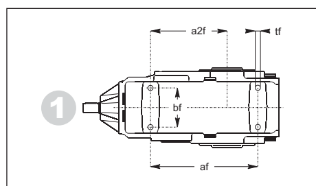
Particolare corpo in versione flangiata / Detail of the flanged gearcase Detail des gehäuses mit abtriebsflansch
